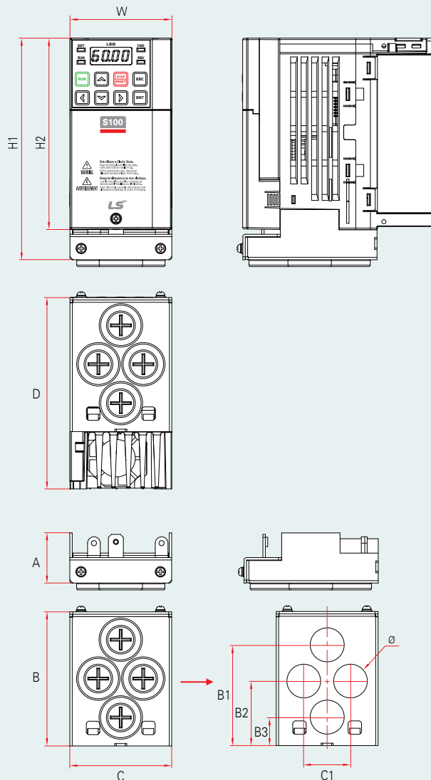
Variador + Conducto
