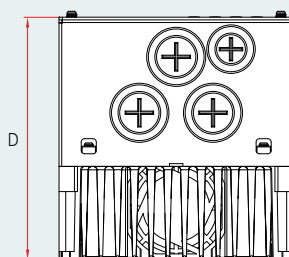
Variador + Conducto
